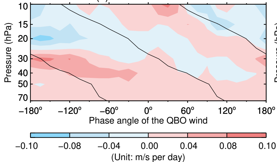
(c) El Niño – La Niña
