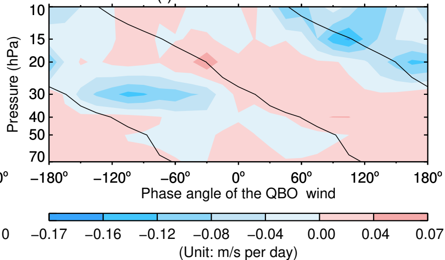
(f) El Niño – La Niña
