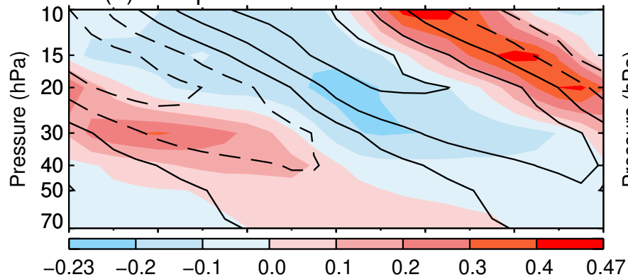
(c) El Niño – La Niña
