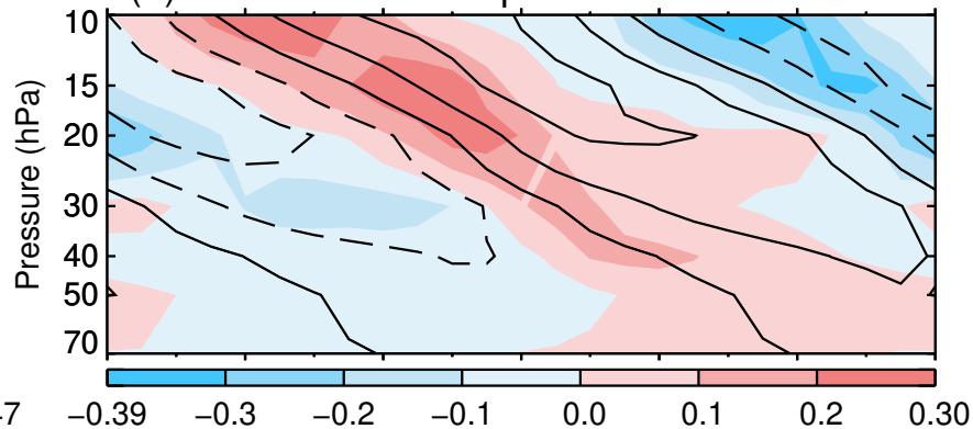
(f) El Niño – La Niña
