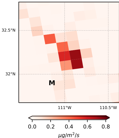
(d) NEI emission E_{NEI}
