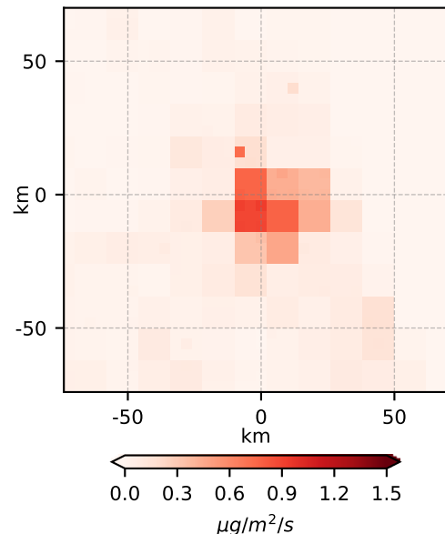
(d) NU-WRF given \text{NO}_x emission E'_{\text{NU-WRF}}
