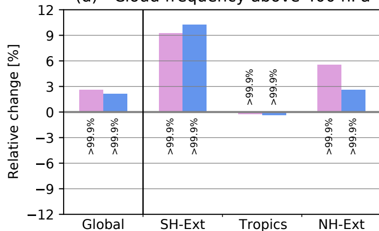
(d) - Cloud frequency above 400 hPa
