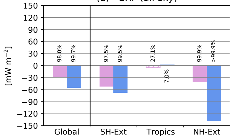
(a) - ERF (all-sky)
