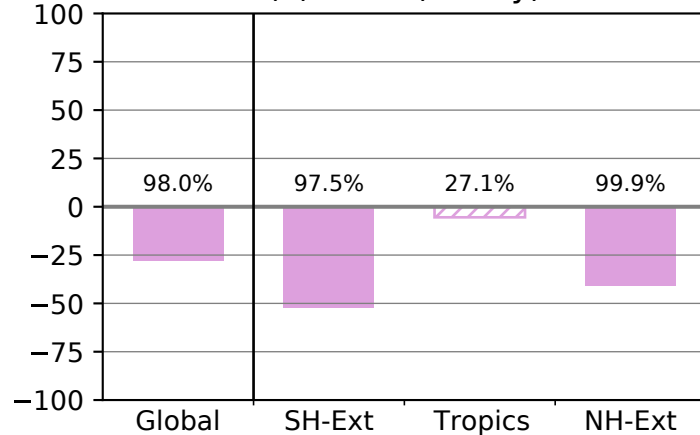
(a) - ERF (all-sky)
