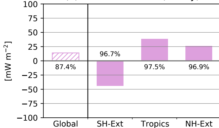
(b) - Shortwave ERF (all-sky)
