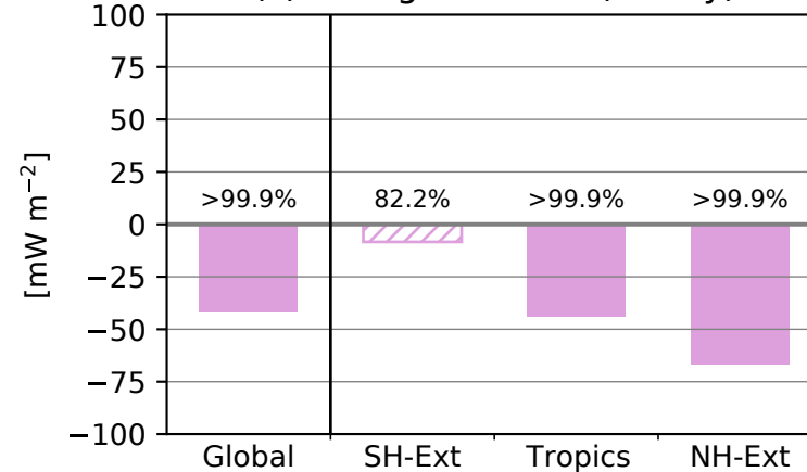
(c) - Longwave ERF (all-sky)
