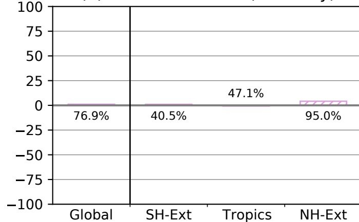
(d) - Shortwave ERF (clear-sky)
