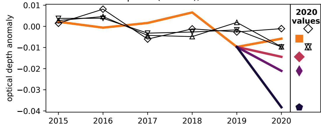
N. Hemisphere (0-70°N), MAM 2015-2020
