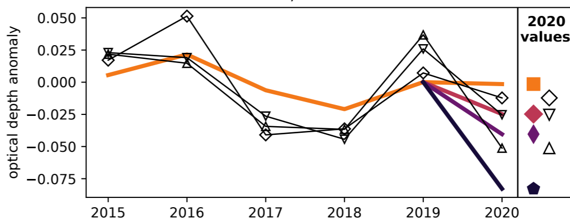
E. China, MAM 2015-2020
