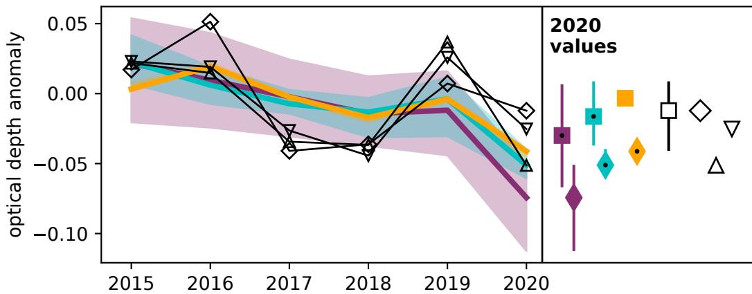
E. China, MAM 2015-2020
