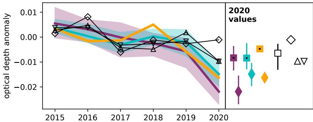
N. Hemisphere (0-70°N), MAM 2015-2020
