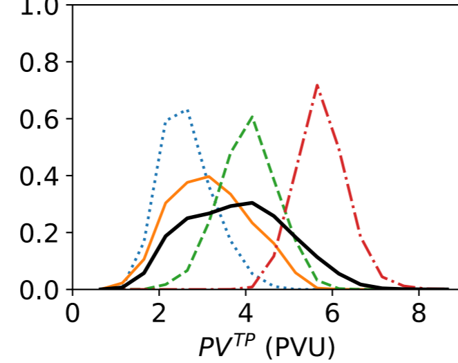
(d) DJF NH, 1D PDFs
