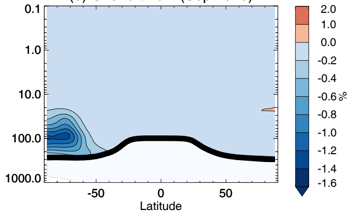
(d) Ozone % diff (Sep 2020)
