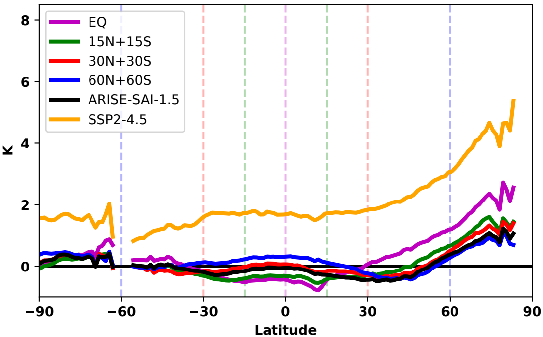
(a) \Delta T_s (land only, 2050-2069)
