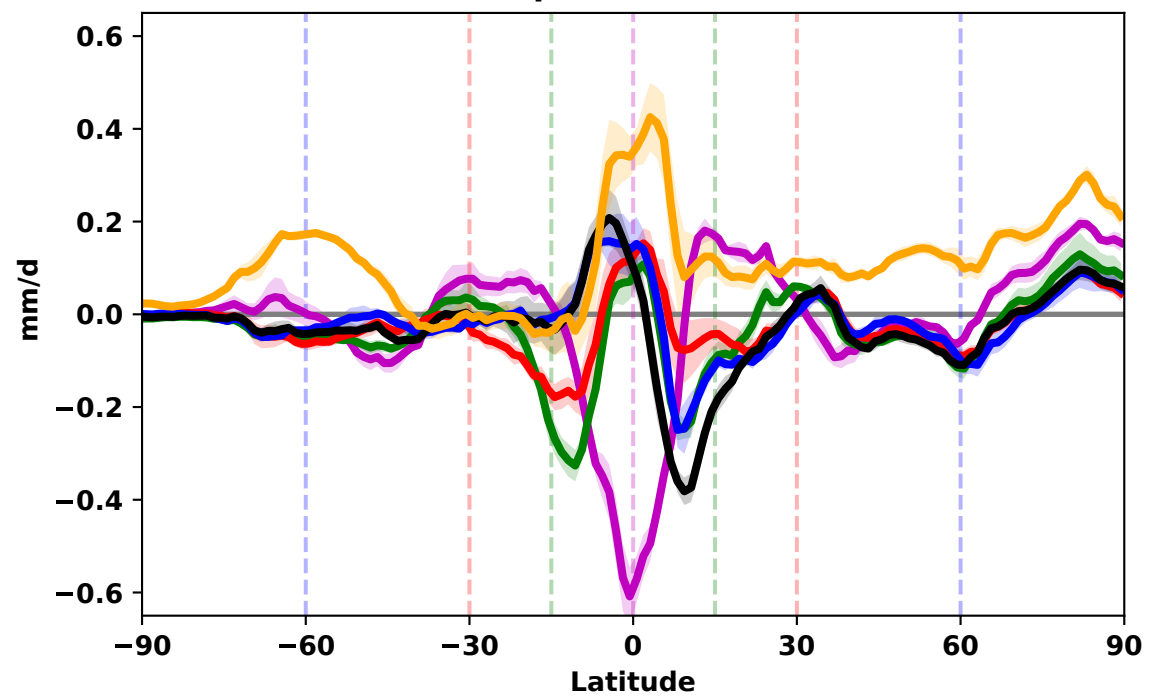
(d) \Delta Precipitation (2050-2069)
