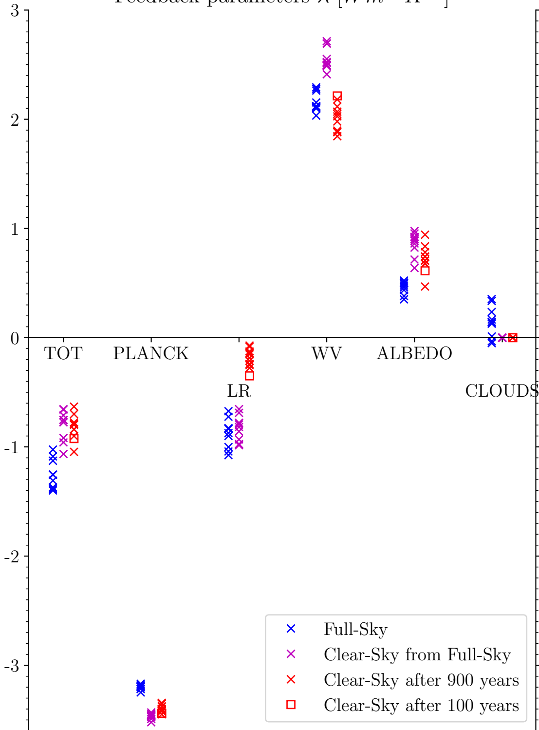
Feedback parameters \lambda [ Wm^{-2}K^{-1} ]
