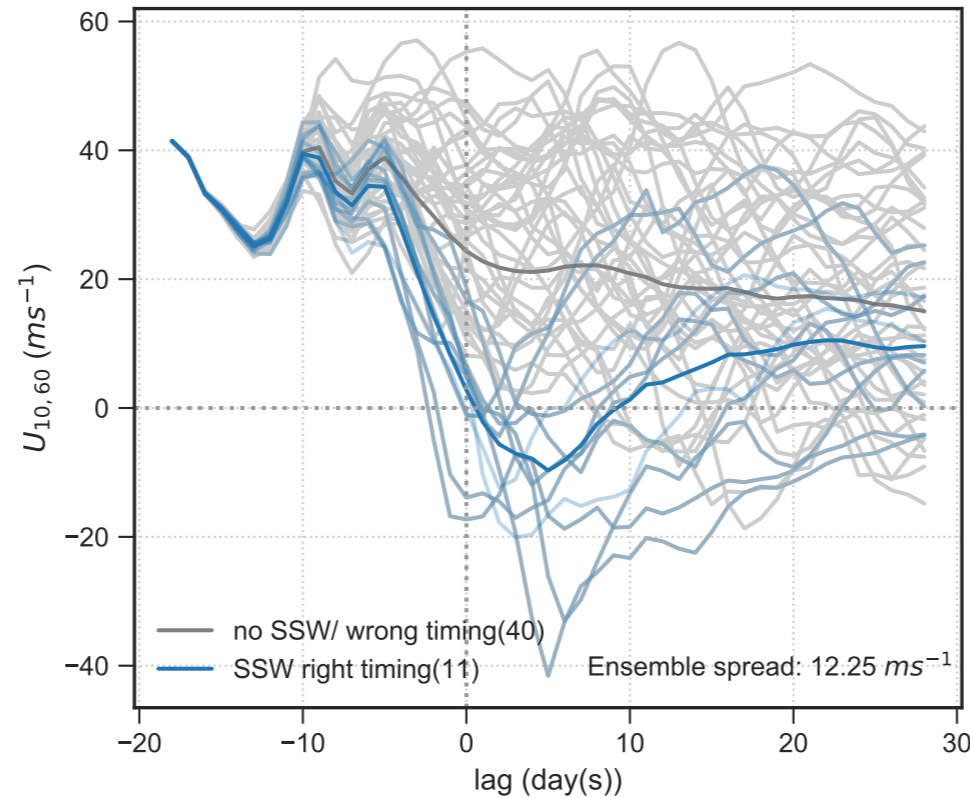
(b) ECMWF hindcast 2018-01-27
