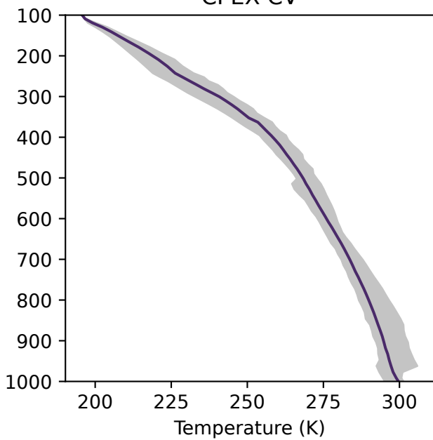
CPEX-CV
