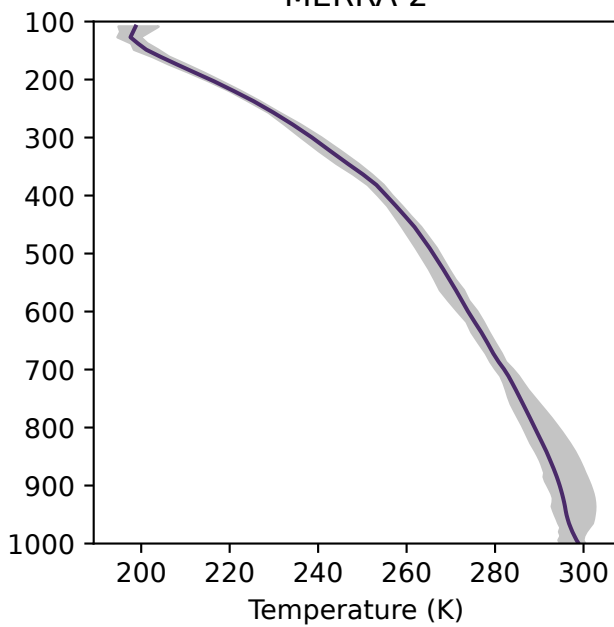
MERRA-2
