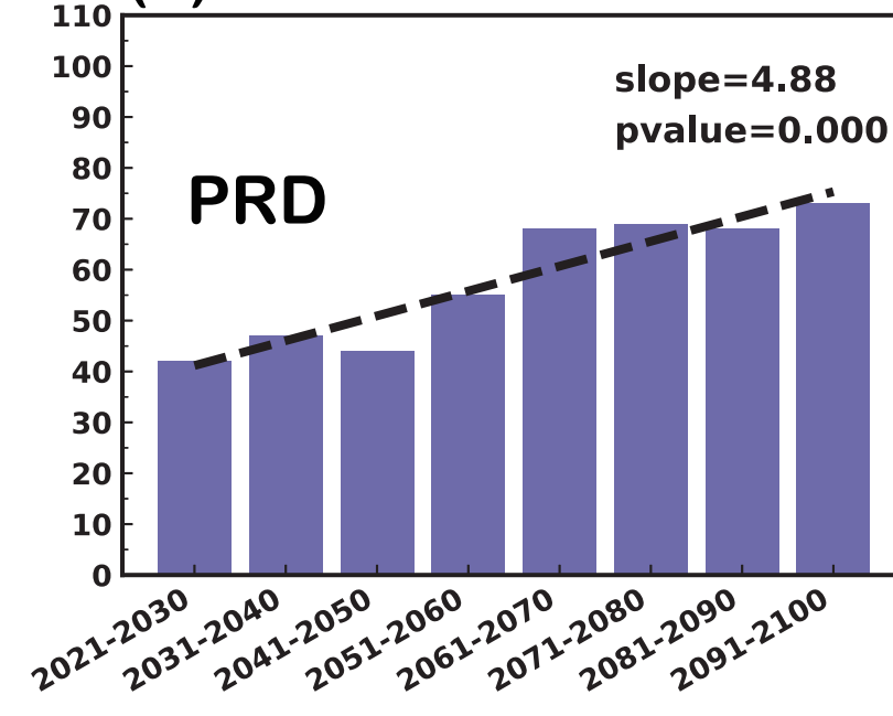
(h) SSP585
