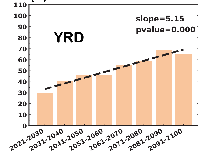
(d) SSP585
