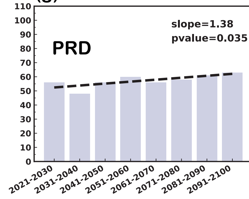
(h) SSP585
