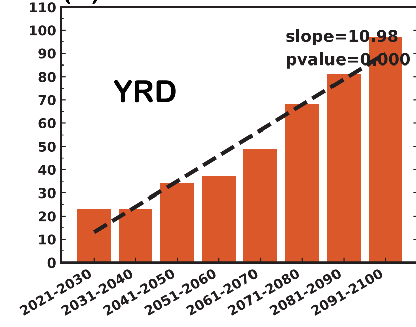
(d) SSP585
