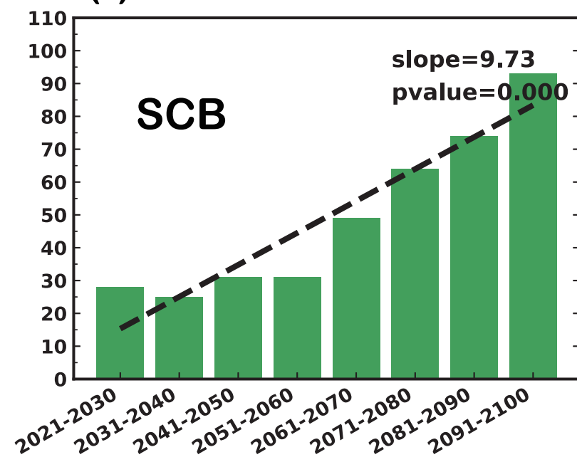
(g) SSP126
