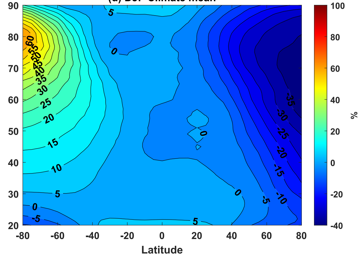
(d) DJF Climate mean
