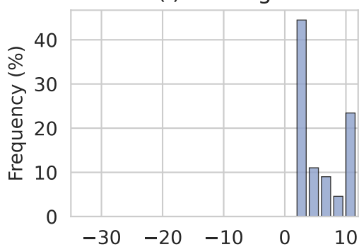
(j) Hom/Het nucl.
