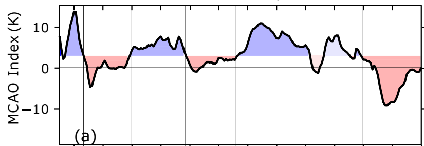
AFLUX: March/April 2019
