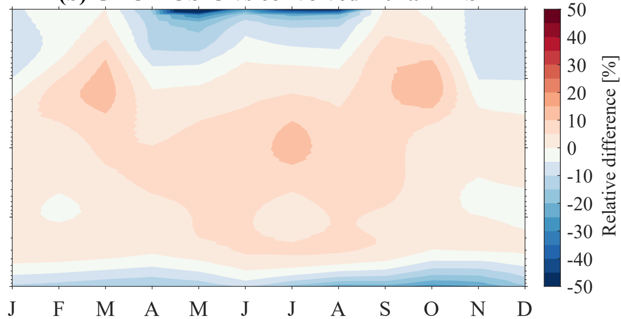
(d) MIAWARA-C vs convolved Aura-MLS
