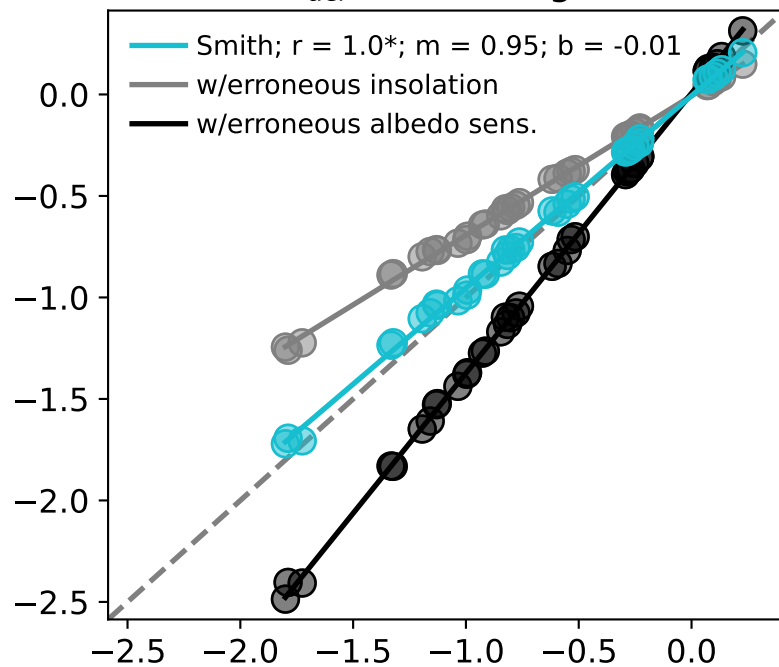
(d) SW ERF aci (absorption)
