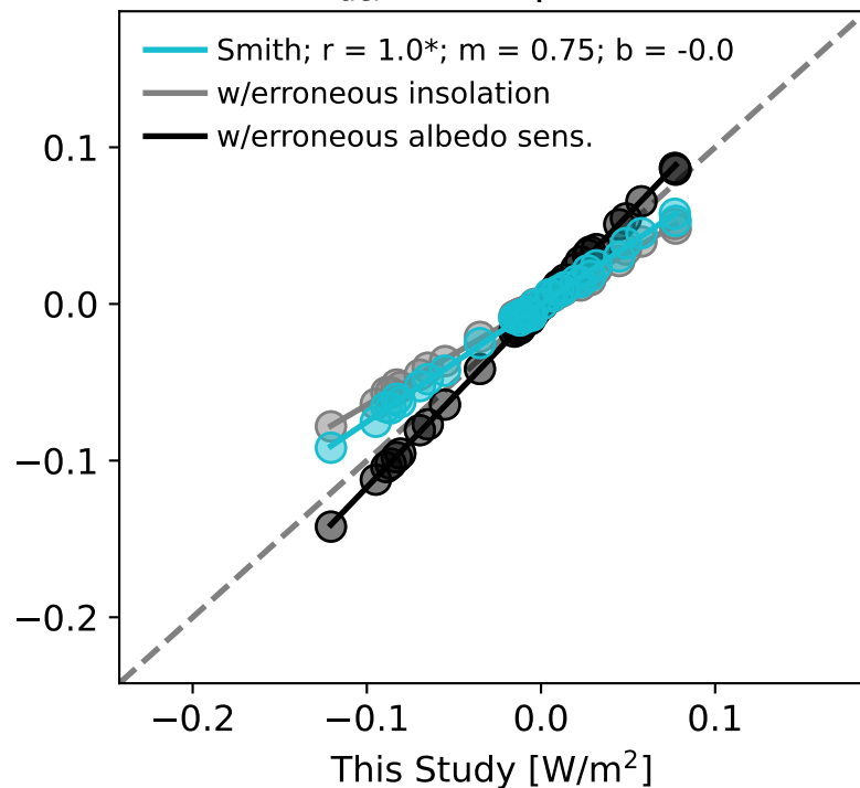
(d) SW ERF aci (absorption)
