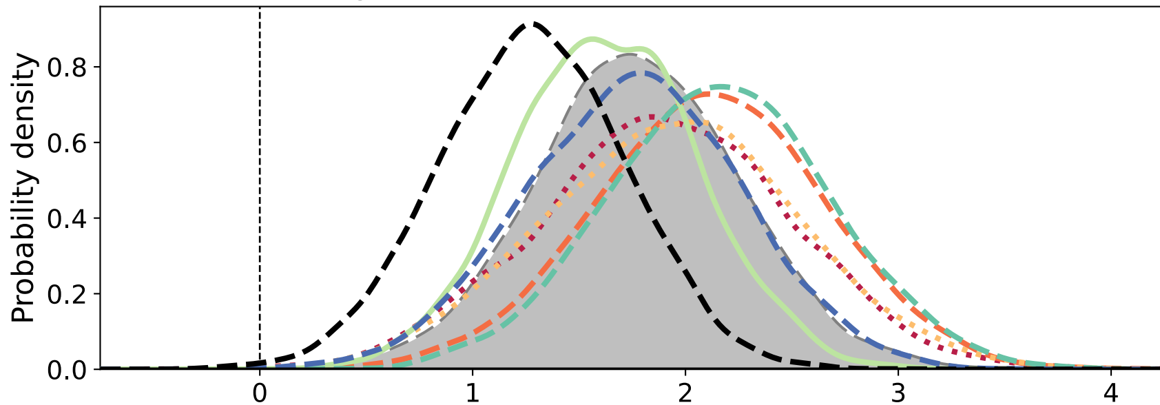
(d) Relative change in annual mean A_{\text{cld}} (%)
