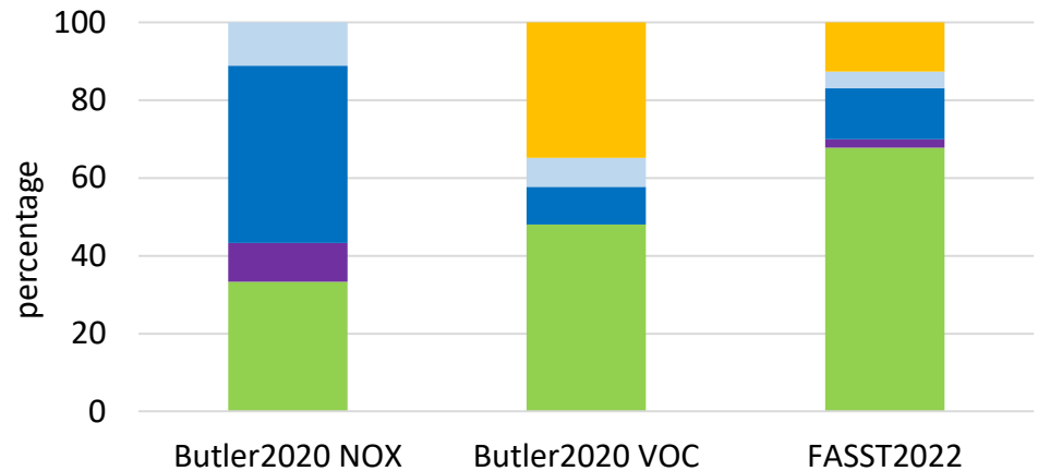
(b) O 3 UNECE SOURCES SUMMMER 2010
