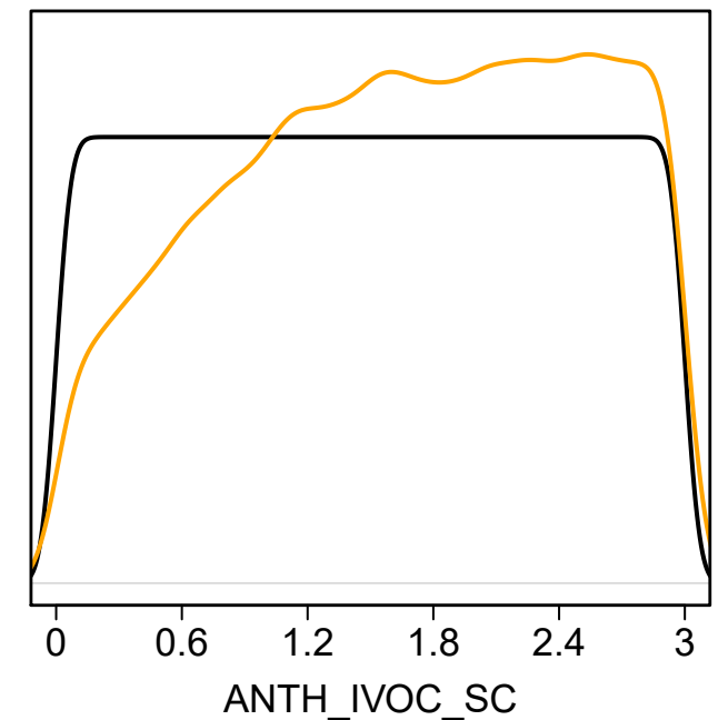
4. ANTH_IVOC_SC
