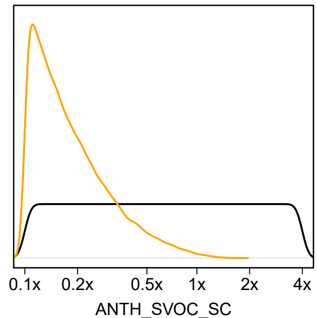
5. ANTH_SVOC_SC
