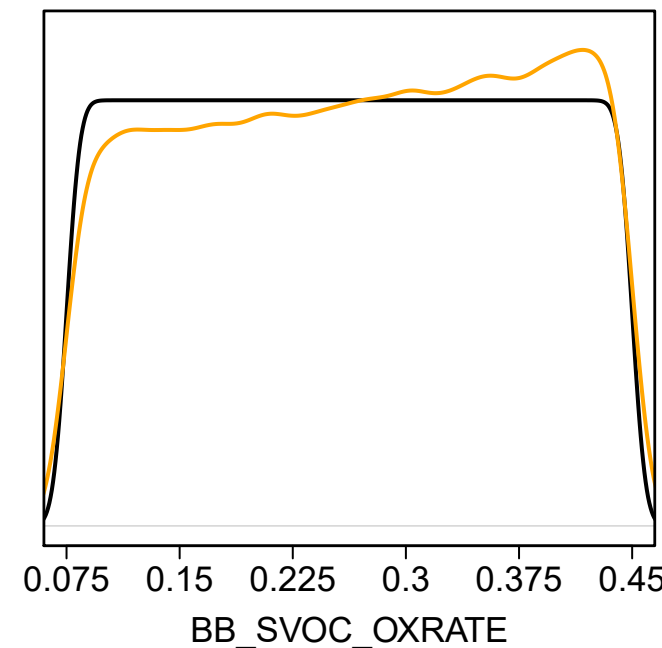
8. BB_SVOC_OXRATE
