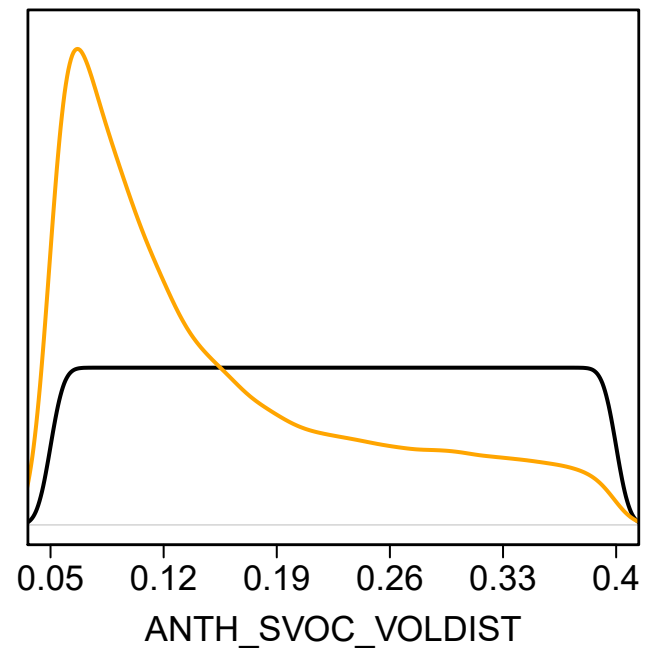
2. ANTH_SVOC_VOLDIST
