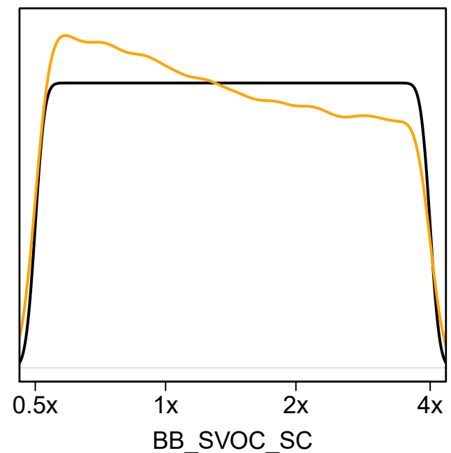
10. BB_SVOC_SC
