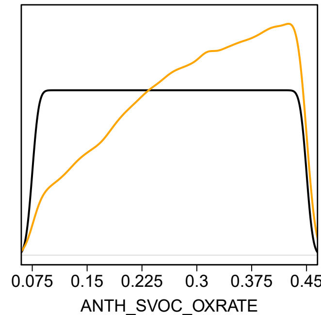
3. ANTH_SVOC_OXRATE
