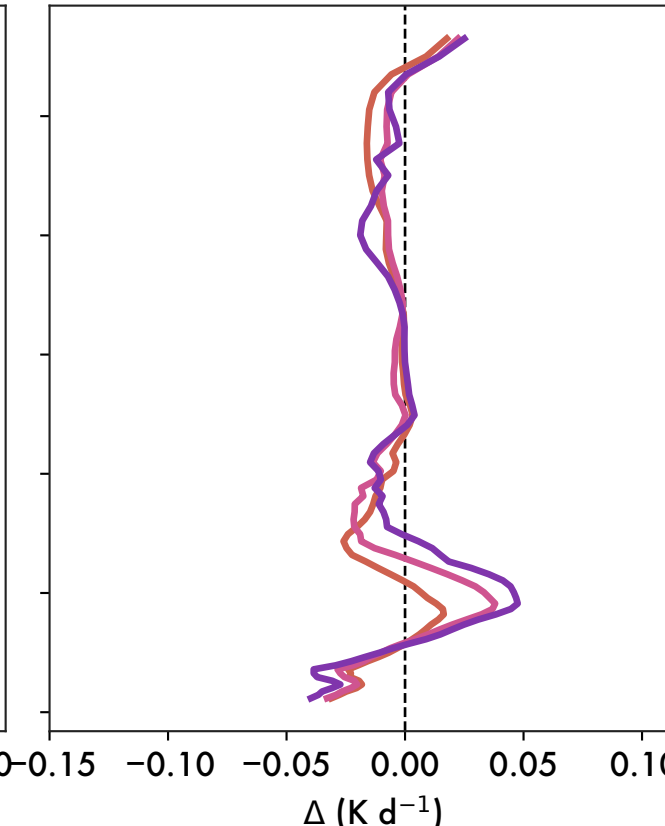
(d) \Delta Mineral Dust
