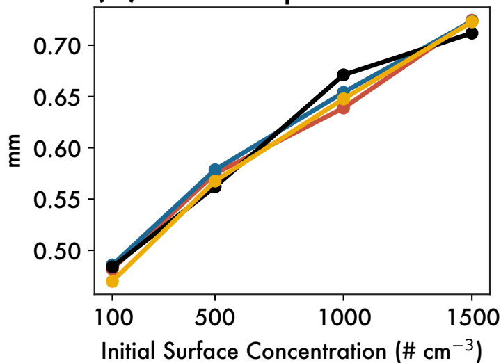
(d) Rain Drop Diameter
