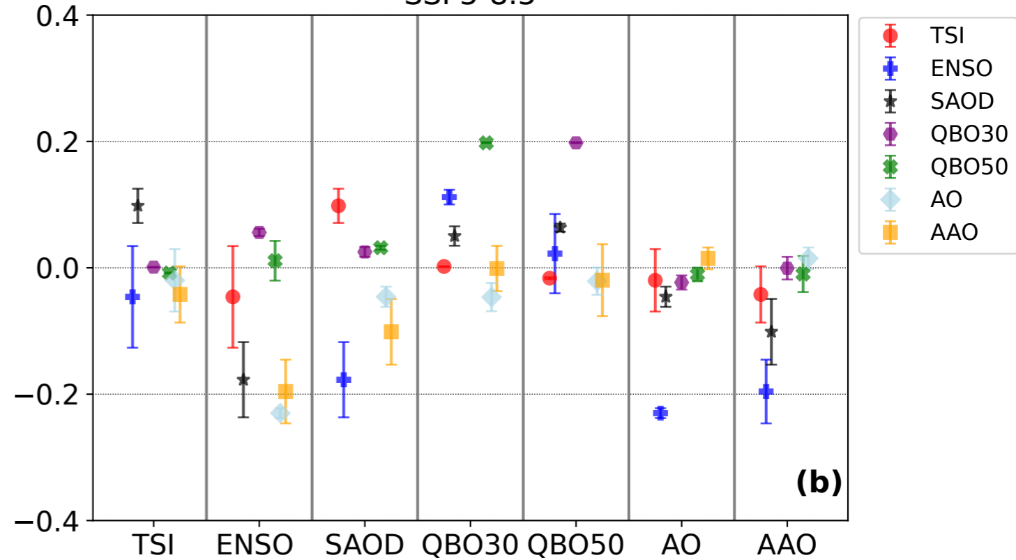
SSP5-8.5
