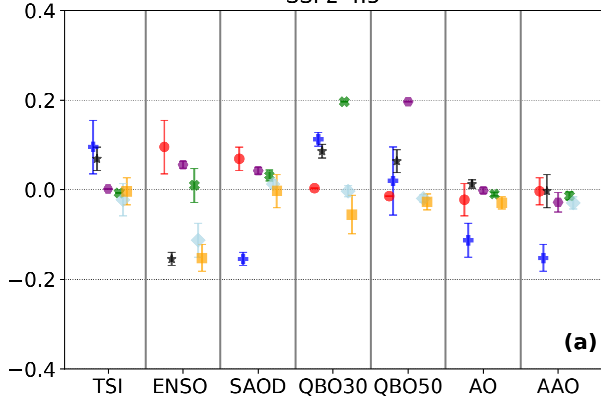
SSP2-4.5
