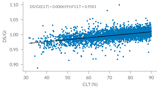
(d) Andøya cloud effect on GI
