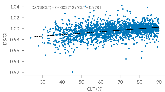
(d) Andøya cloud effect on GI
