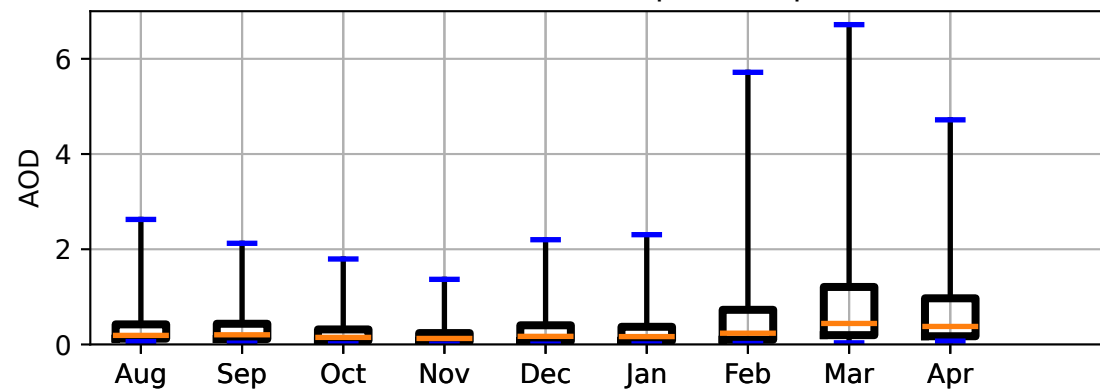
(d) AH - Aerosol optical depth
