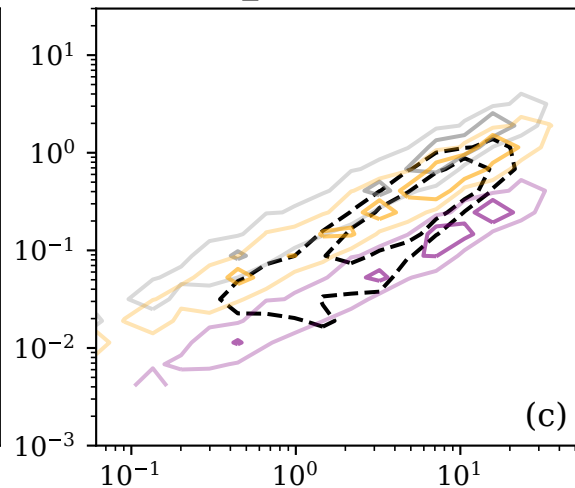
integ. IWC ( \text{kg m}^{-2} )
