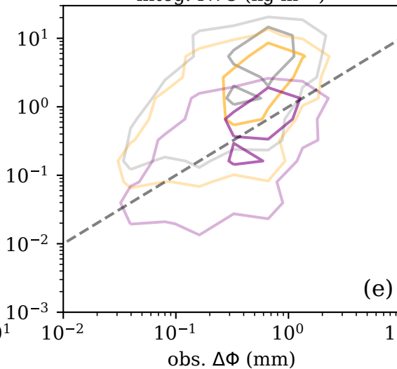
integ. IWC ( \text{kg m}^{-2} )
