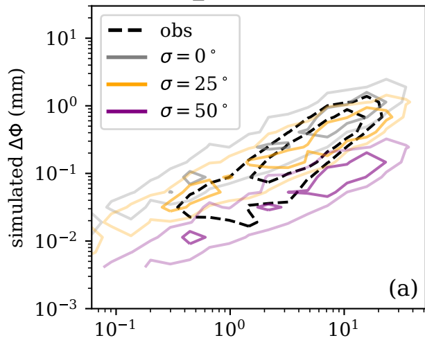
integ. IWC ( \text{kg m}^{-2} )
