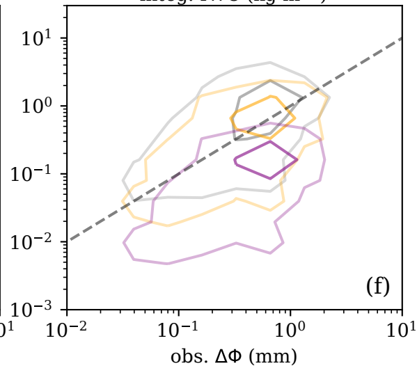
integ. IWC ( \text{kg m}^{-2} )
