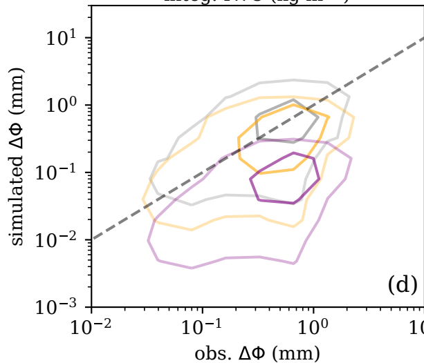
integ. IWC ( \text{kg m}^{-2} )
