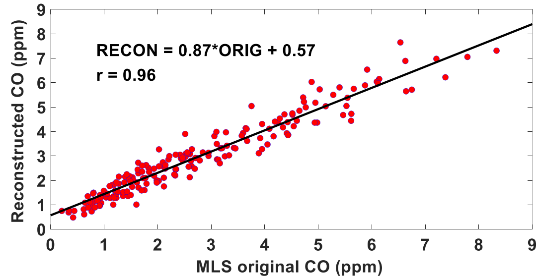
(d) MLS original VS reconstructed CO at ~90 km
