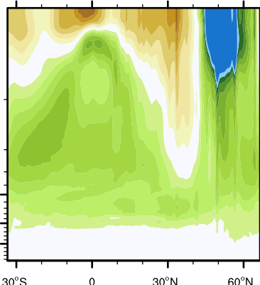
(d) ARISE-SAI-1.5
