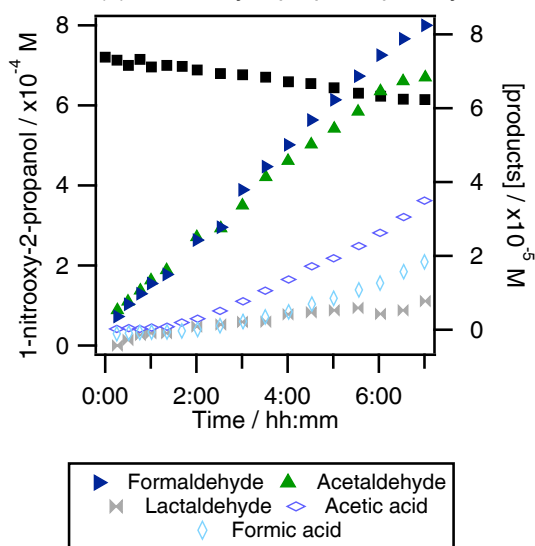
(d) 1-Nitrooxy-2-propanol photolysis
