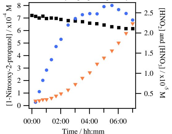
(d) 1-Nitrooxy-2-propanol photolysis
