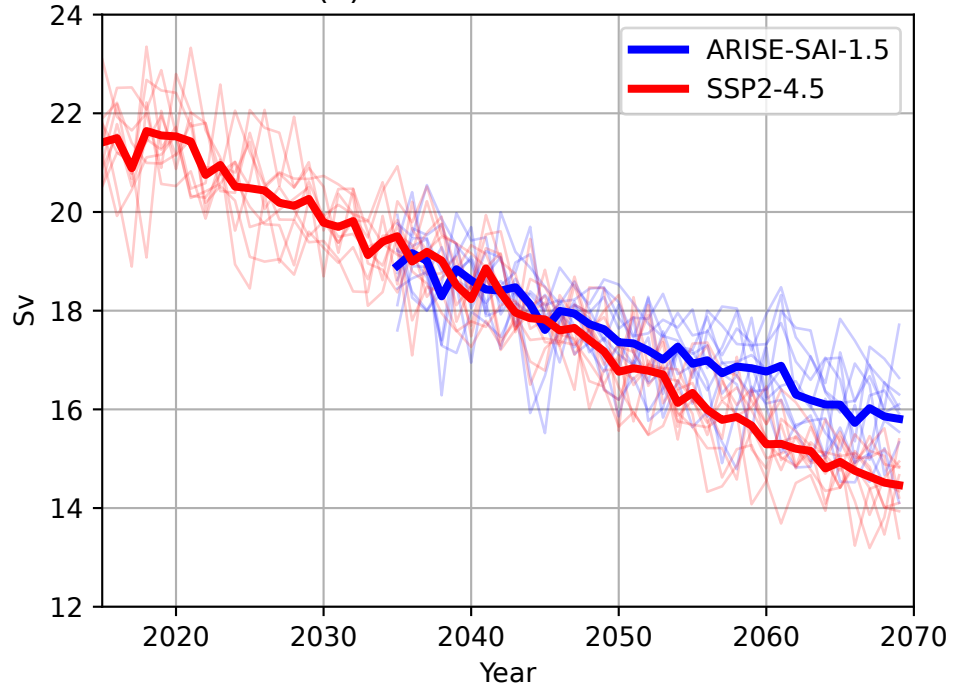
(b) CESM2 Atlantic MOC
