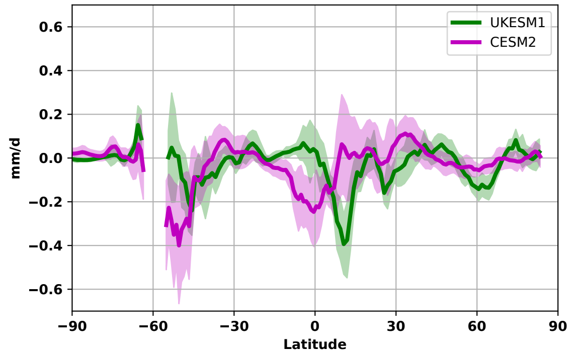
(d) Land precipitation (ARISE-SAI-1.5, JJA, 2050-2069 - reference period)
