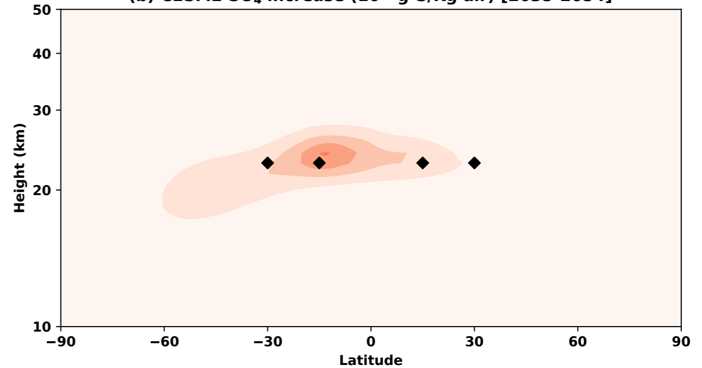
(d) CESM2 SO 4 increase (10 -9 g-S/Kg air) [2050-2069]
