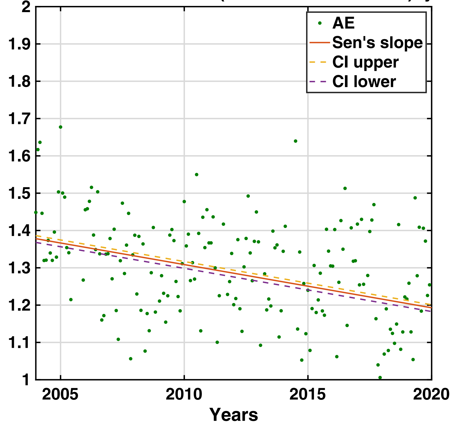
AE @440-870nm -0.011(CI 95%:-0.017 -0.0075) yr -1
