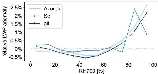
(d) LWP enhancement by RH700 bins
