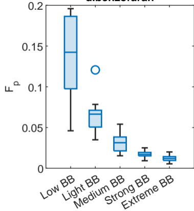
dibenzofuran
