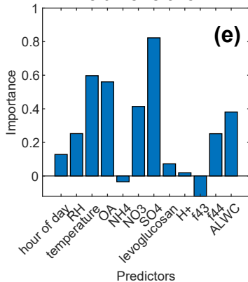
C5 alkene triol-1
