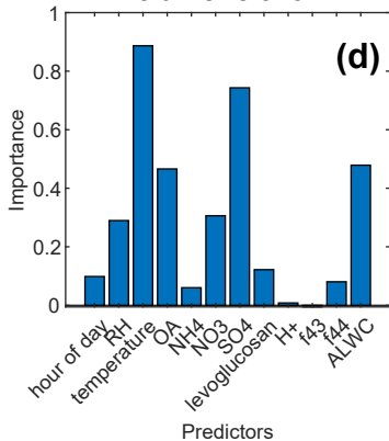
C5 alkene triol-2
