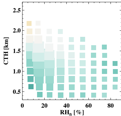
(e) NE Atlantic
