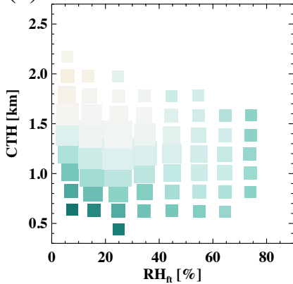
(d) SE Atlantic
