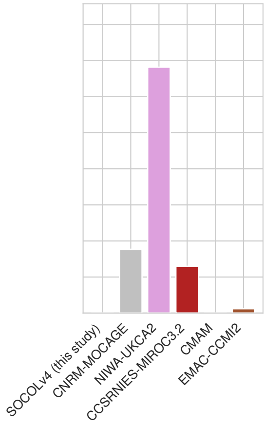
SSP2-4.5 - CCMI-2022
