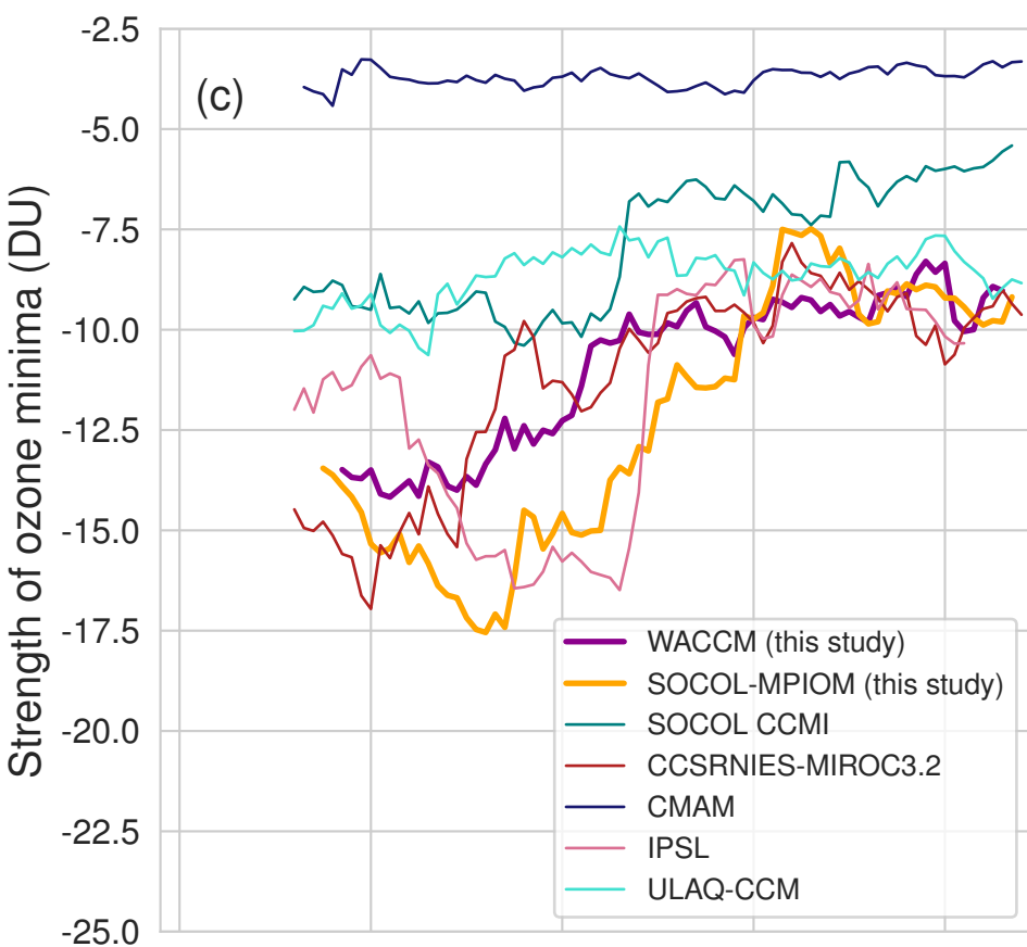
SSP2-4.5 - CCMI-2022
