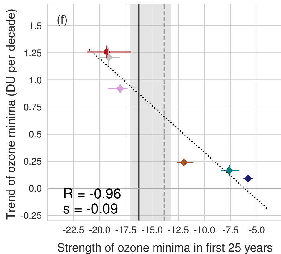
SSP2-4.5 - CCMI-2022
