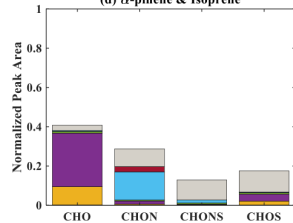
(d) \alpha -pinene & Isoprene
