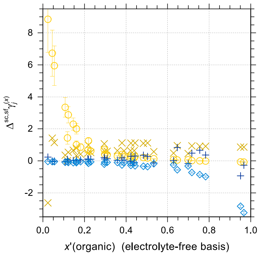
(a) H 2 O (1) + Acetone (2) + KI (3)
