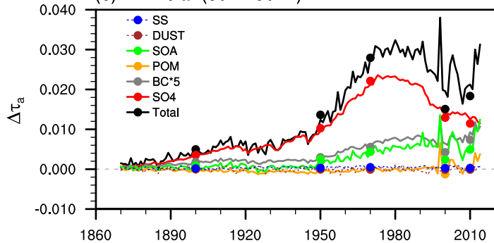
(d) Tropics (20°S-20°N)
