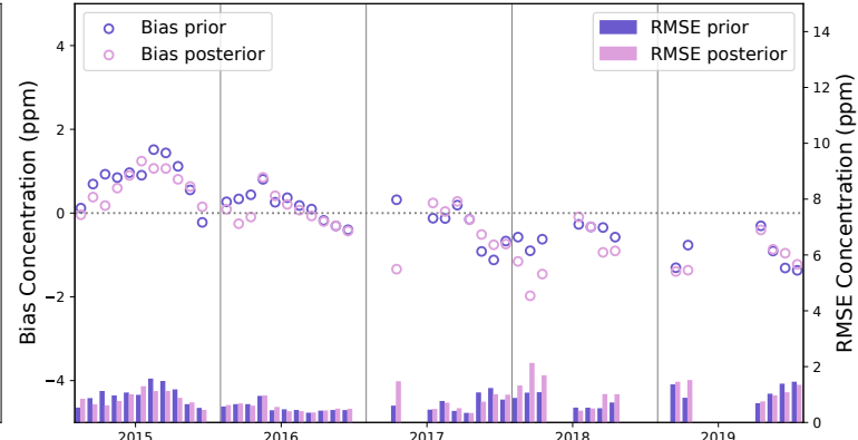
(d) Bias and RMSE Wollongong
