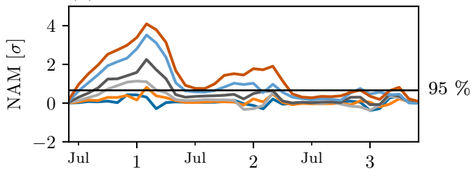
(b) 100 hPa
