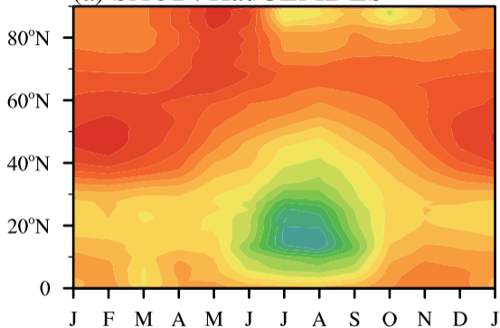
(a) SAOD: HadGEM2-ES
