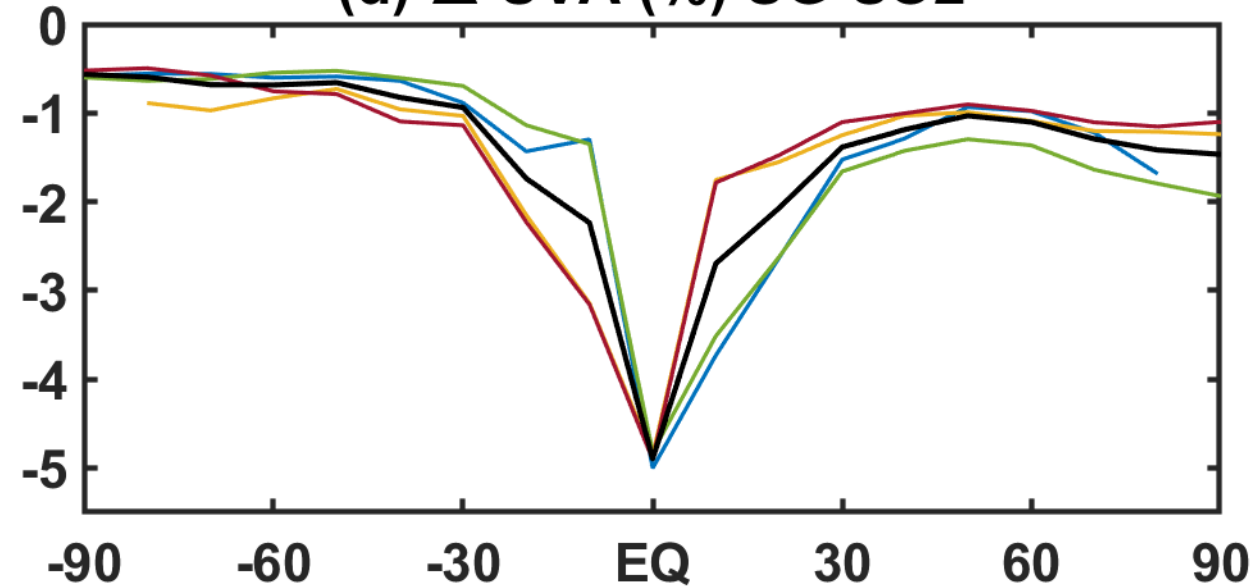
(d) \Delta UVA (%) SG-SO2
