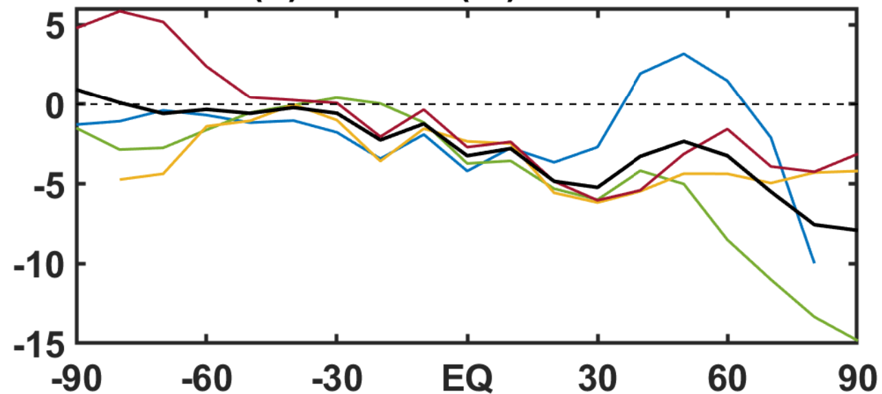
(b) \Delta UVB (%) SG-SO2
